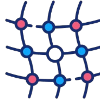
Chaos Mesh
